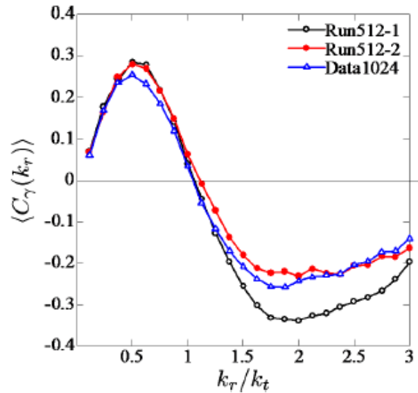
図 5 渦のスケールと伸長速度
