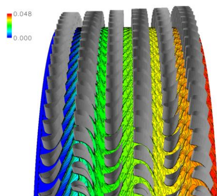
(a) ミッドスパン
