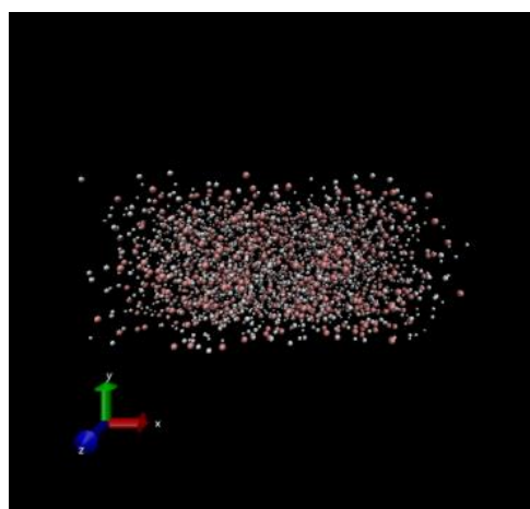
図 3 引張シミュレーション前
