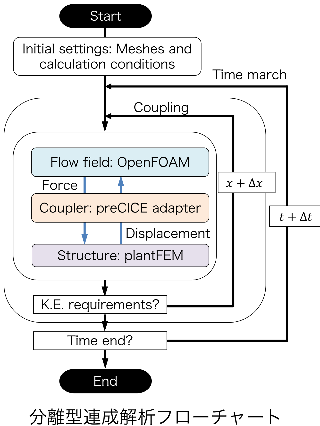
分離型連成解析フローチャート
