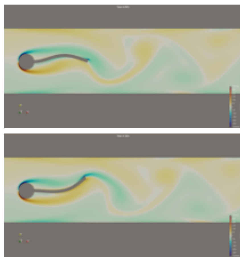
preCICEを用いたFSIシミュレーションの一例 (Turek-Hron FSI case)
