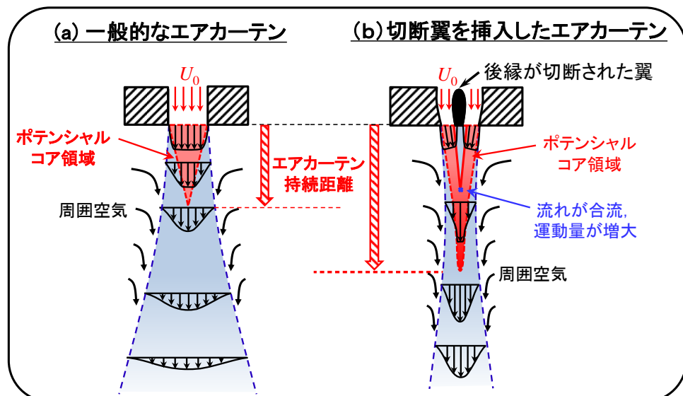
図1: エアカーテンの性質比較の概要図
