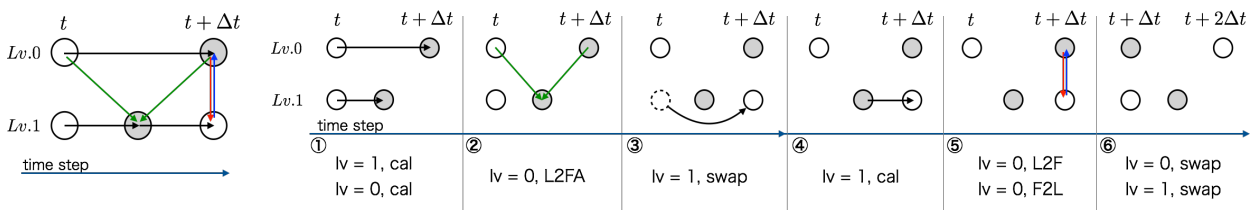
図 1 AMR 法を適用した LBM での計算順序例。①LBM 計算、②Lv.1 への時空間補間、③Lv.1 での swap、④Lv.0 と Lv.1 での空間補間、⑤Lv.0 と Lv.1 での swap、以後①～⑤の繰り返し。②および⑤は解像度が異なる領域と重なる Halo 領域に対しての更新する。
