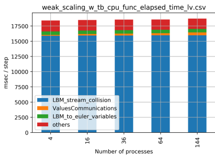
図 5 テンポラルブロッキング法を採用した CPU 計算での弱スケーリング結果(4MPI Procs/node)
