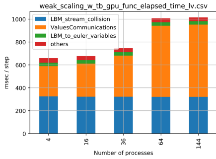
図 3 テンポラルブロッキング法を採用した GPU 計算での弱スケーリング結果
