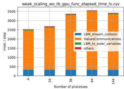
図 4 テンポラルブロッキング法無しの GPU 計算での弱スケーリング結果
