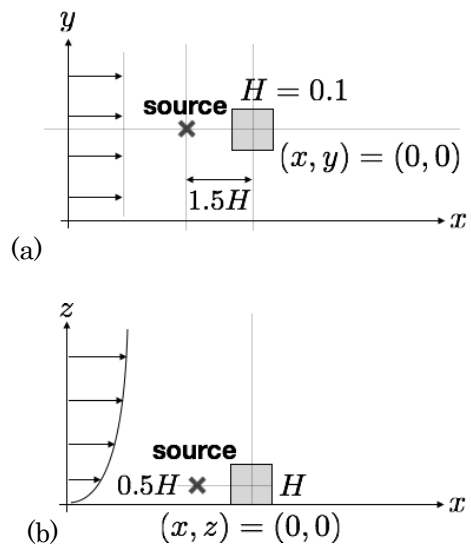
図 6 産総研の風洞実験に対する計算条件
