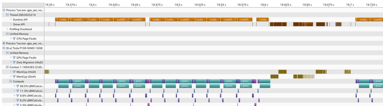
図 2 テンポラルブロッキング法を採用した LBM での Nvprof を用いたタイムラインの可視化 (4MPI プロセス、AMR:Lv.0 ~ Lv.2、Leaf size=8)
